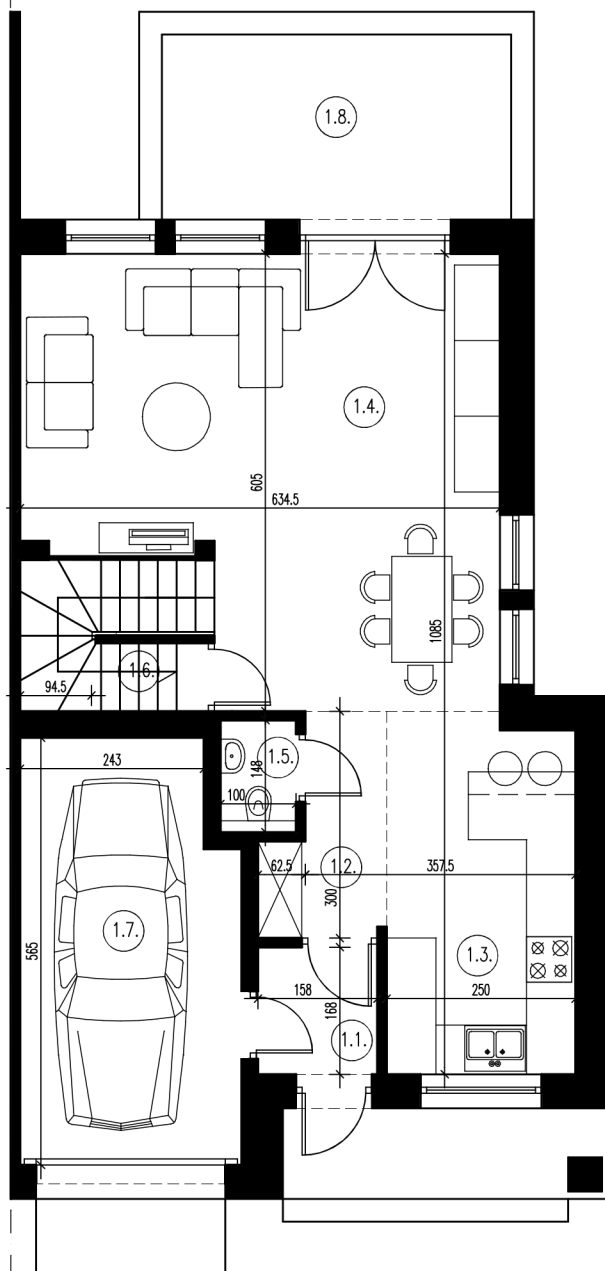
RZUT PARTERU
