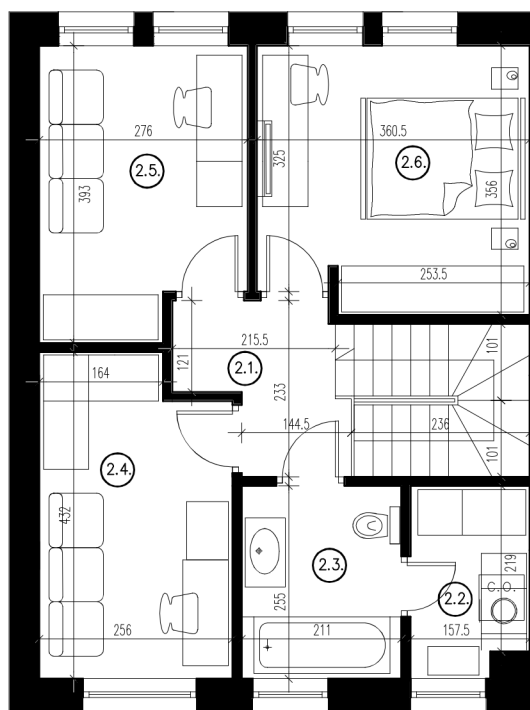
RZUT PIĘTRA
